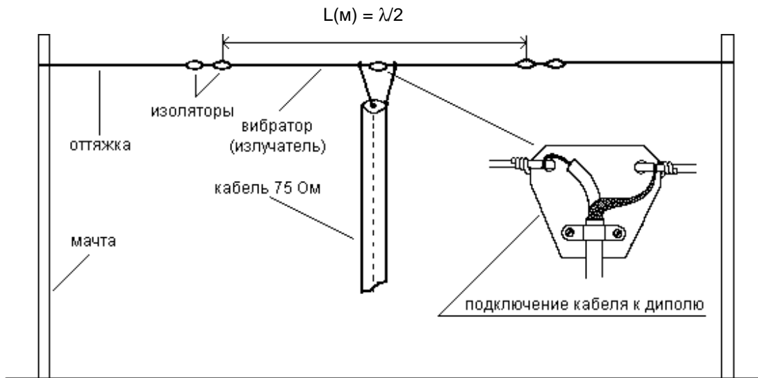
Рис.2.9. Антенна «диполь»
