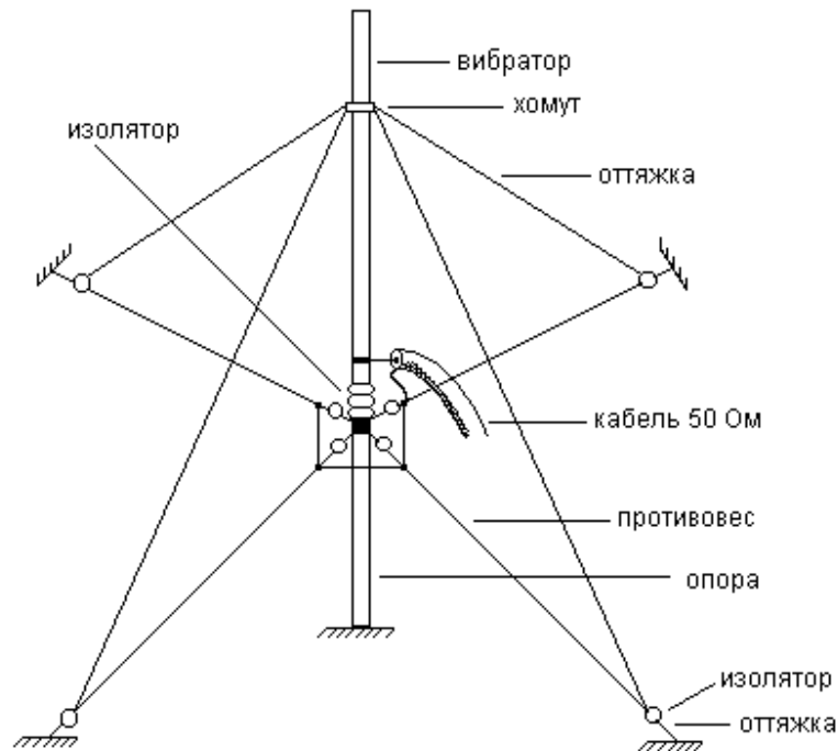
Рис.2.12. Антенна «граунд-плэйн»
