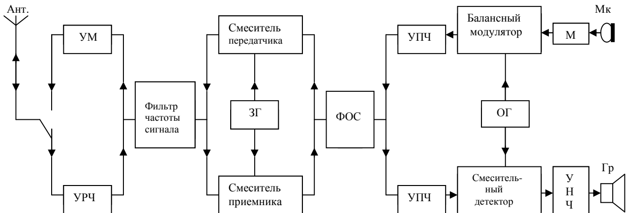
Рис. 2.3. Структурная схема SSB-трансивера
